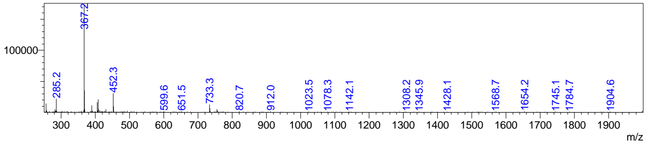
MS Spectrum(KAB8-2_2.lcd)
