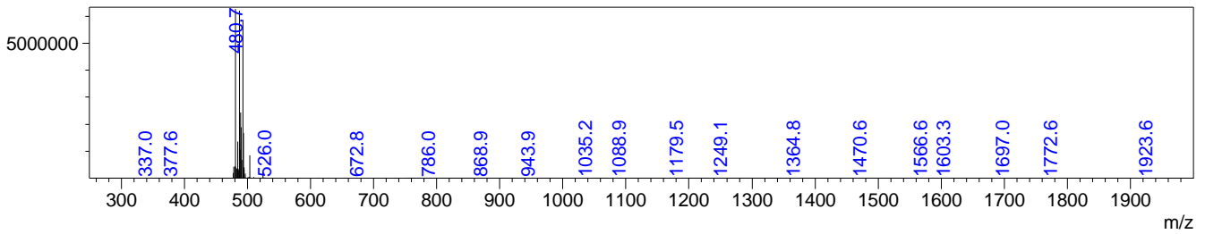
MS Spectrum(MNR11-8.lcd)
