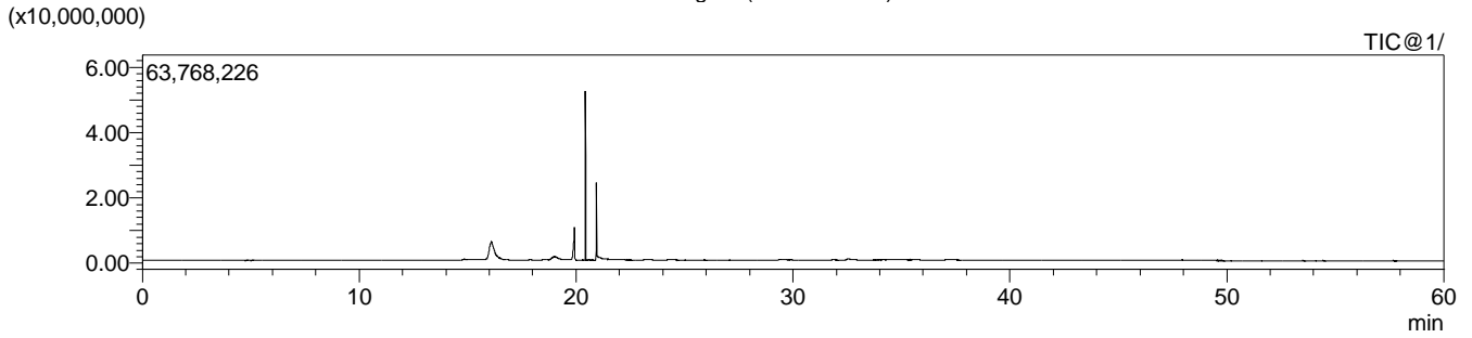
MS Spectrum(MNR11-8.lcd)
