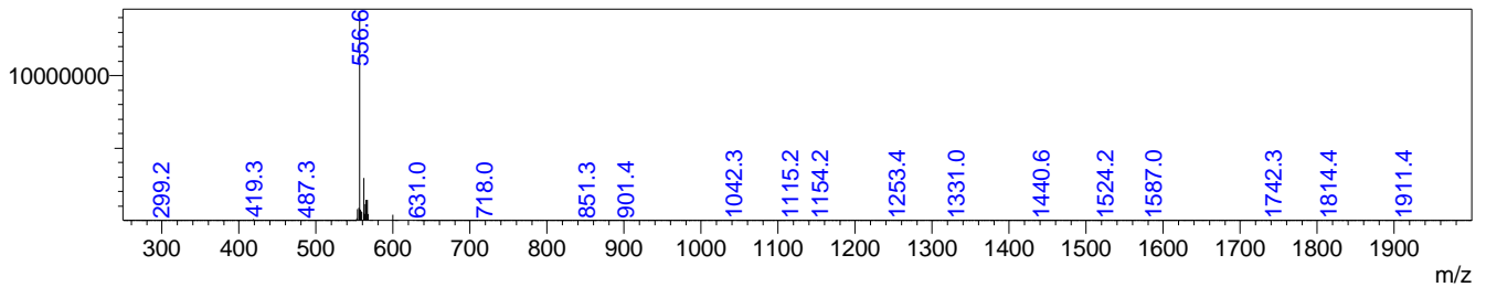
MS Spectrum(MNR11-8.lcd)
