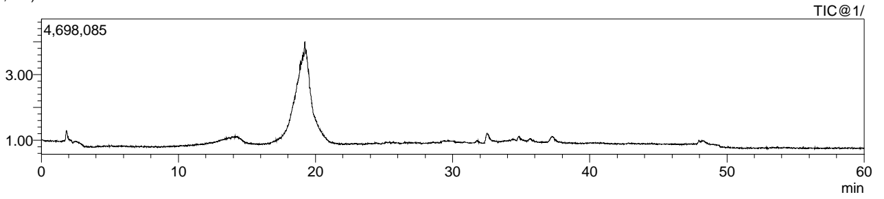
MS Spectrum(MNR11-7.lcd)
