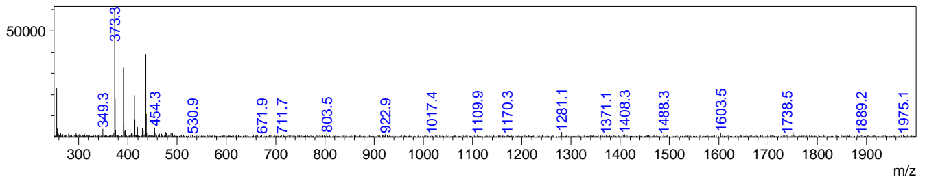
MS Spectrum(MNR11-7.lcd)
