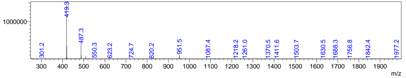
MS Spectrum(MNR11-7.lcd)
